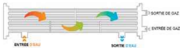
SYSTÈME MULTITUBULAIRE
