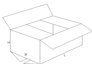
fefco 201
